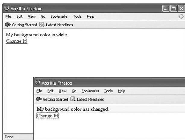
FIGURE 21.1 Using XOAD_HTML::getElementById().
