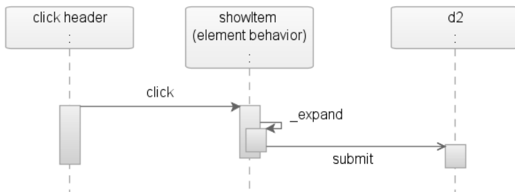
Figure 9-7. HTC <pro:showItem> _expand function
