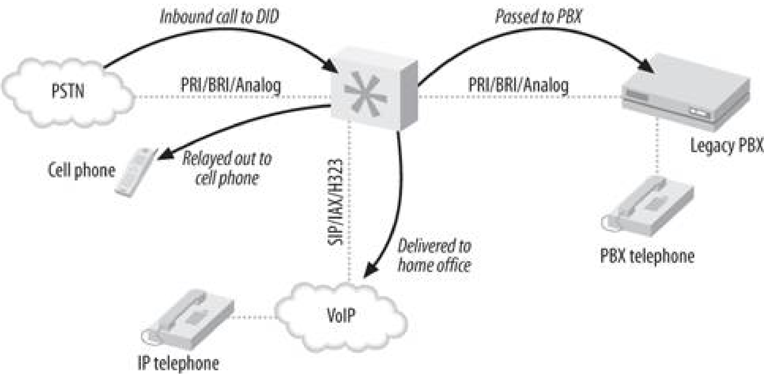
Figure 11-2. Find-me-follow-me
