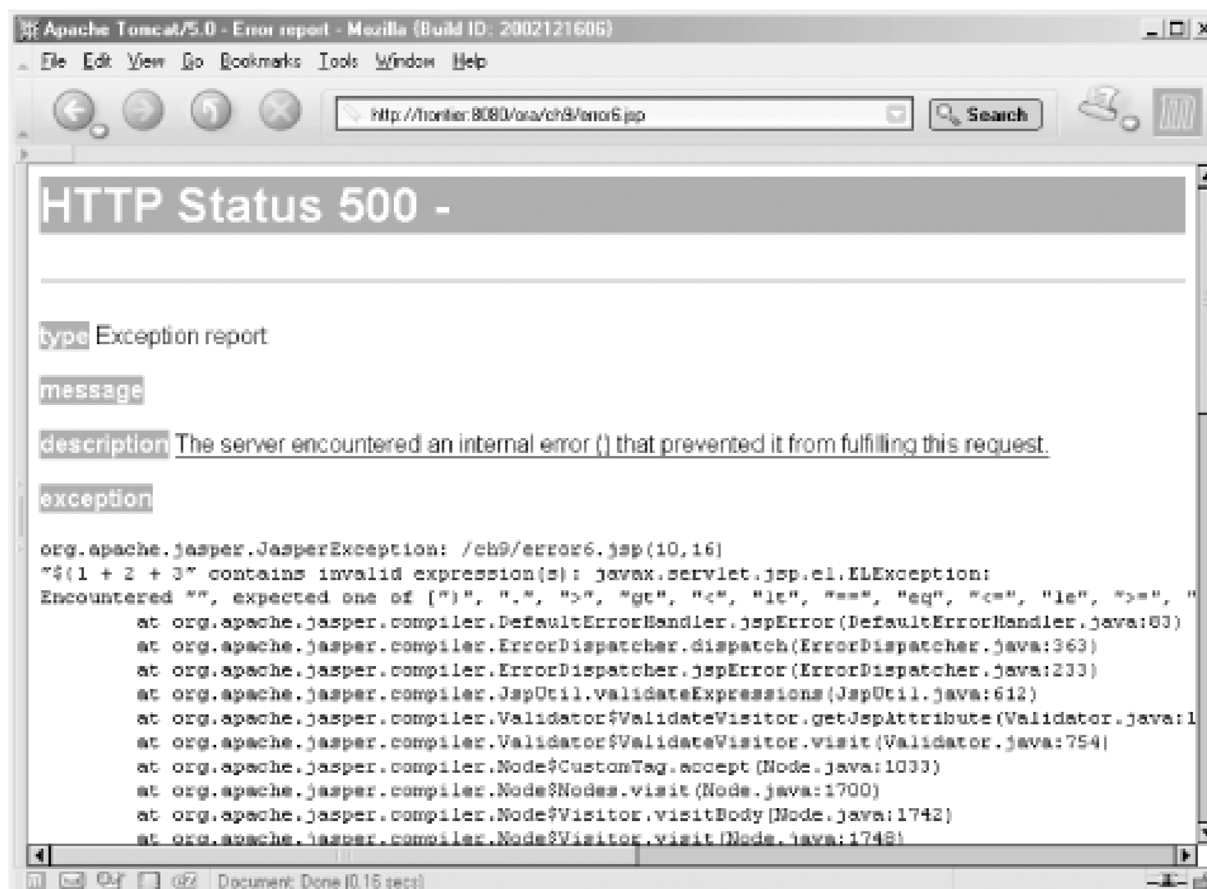
Figure 9-2. EL syntax error message
